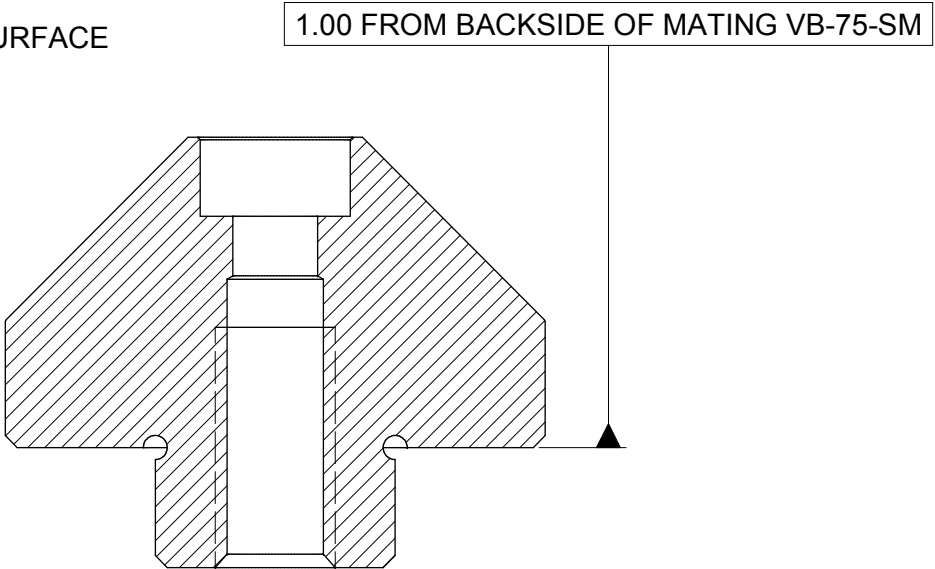
SECTION A-A SCALE 5 : 1
